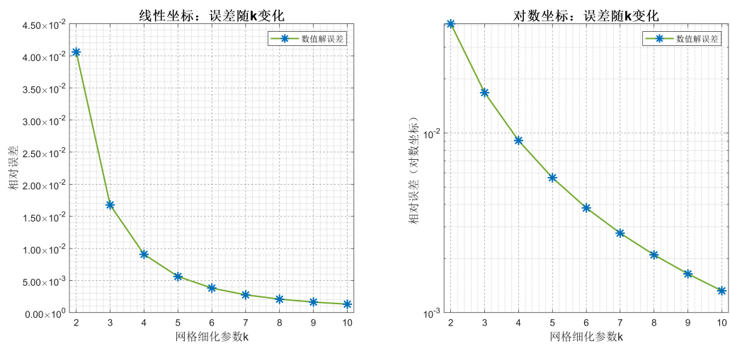
图2 三维有限元误差分析
